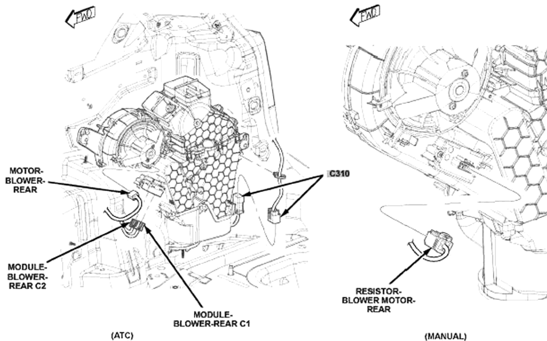
Fig. 33: Right Quarterpanel
