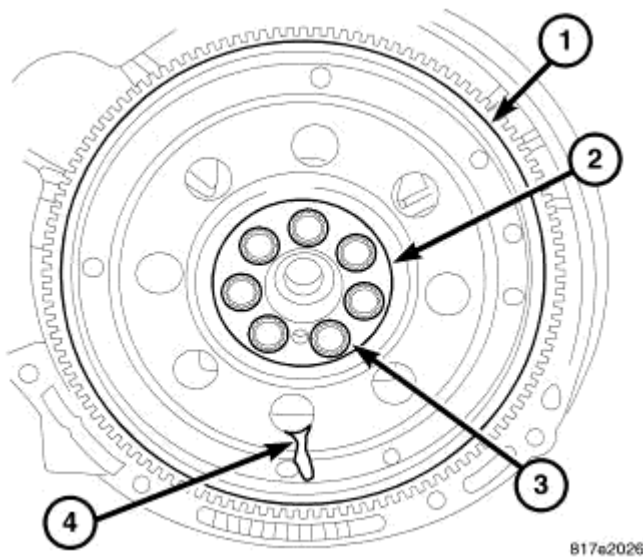
Fig. 199: FLEX PLATE
