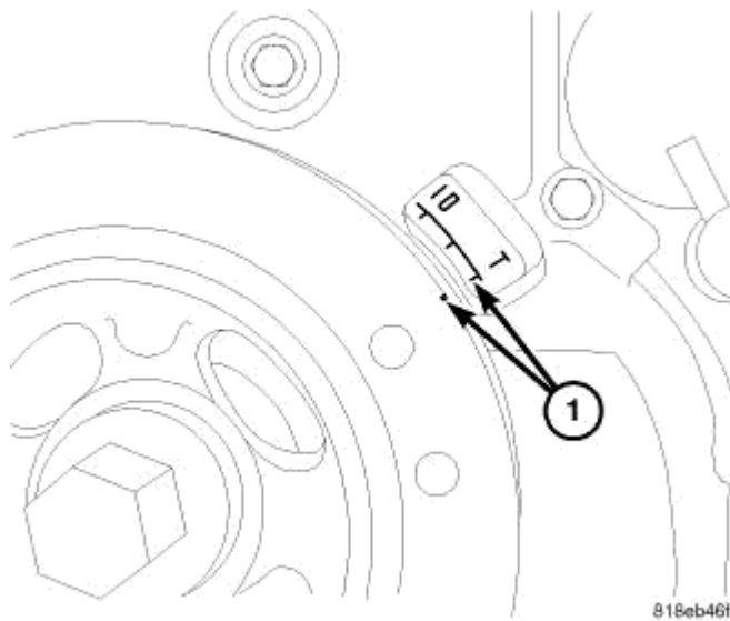
Fig. 126: Top Dead Center
