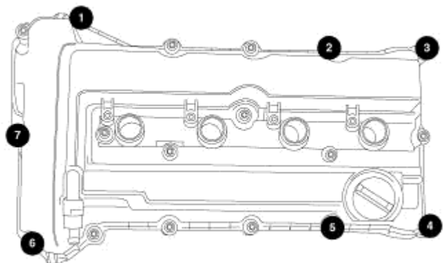
Fig. 154: STUD LOCATION
