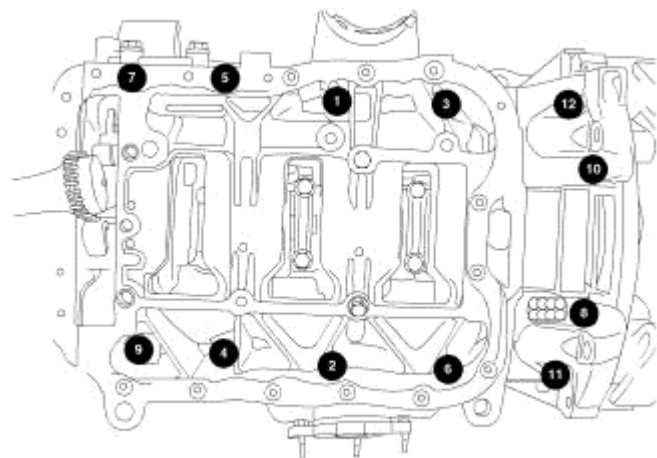
Fig. 203: LADDER FRAME TORQUE
