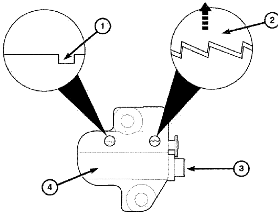
Fig. 394: TENSIONER RESET
