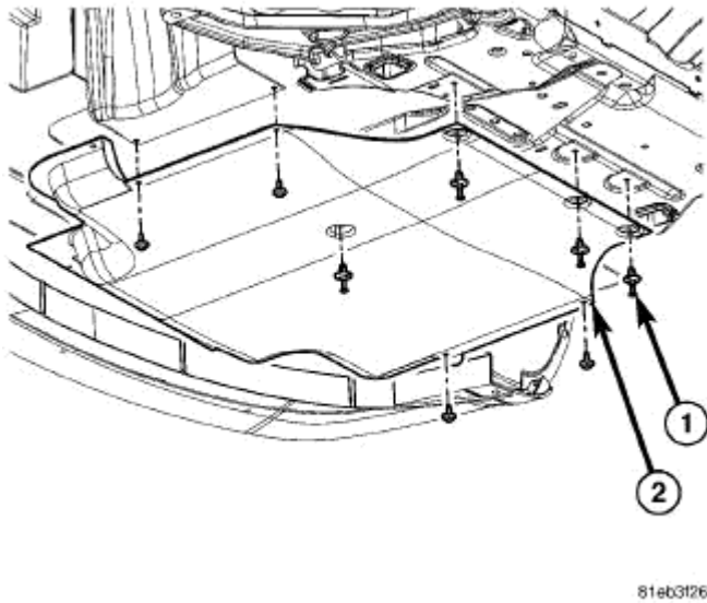
Fig. 273: Belly Pan
