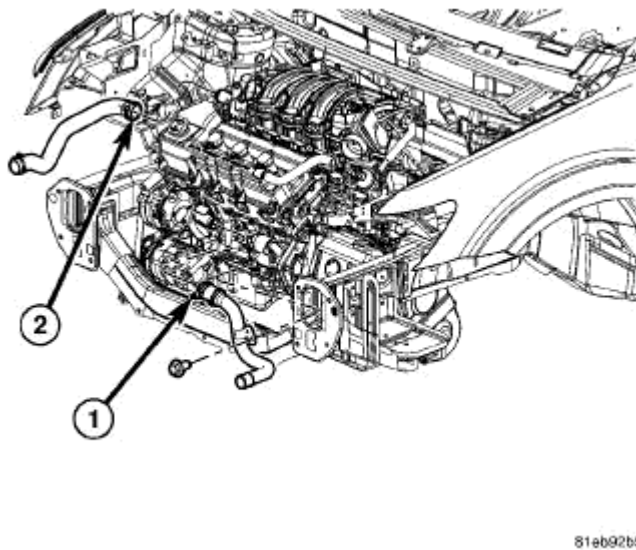
Fig. 50: Upper/Lower Radiator Hoses
