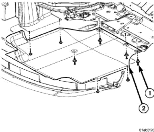
Fig. 287: Belly Pan
