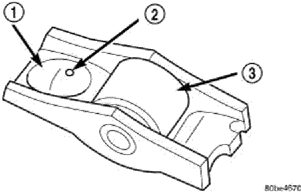
Fig. 133: Rocker Arm
