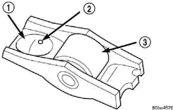
Fig. 136: Rocker Arm
