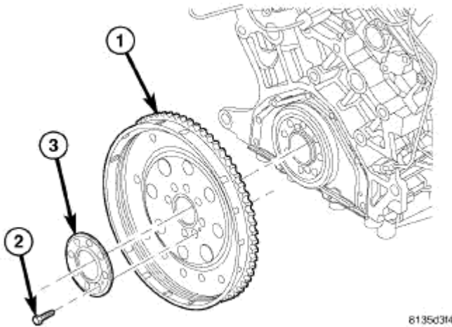
Fig. 215: Flex Plate
