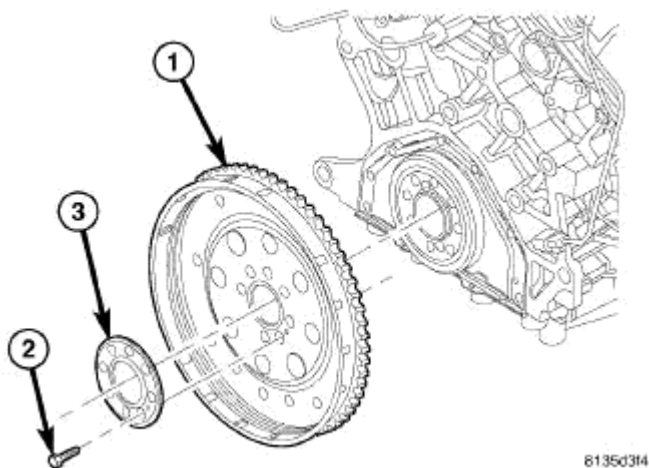
Fig. 198: Flex Plate
