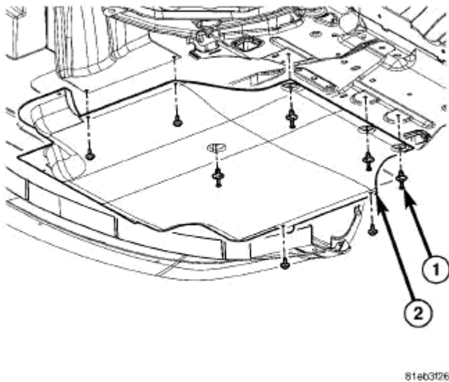
Fig. 316: Belly Pan
