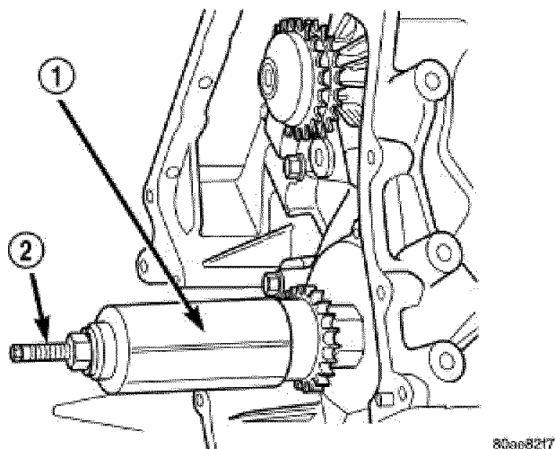
Fig. 347: Crankshaft Sprocket - Installation
