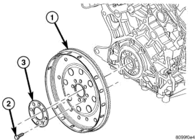
Fig. 199: FLEX PLATE
