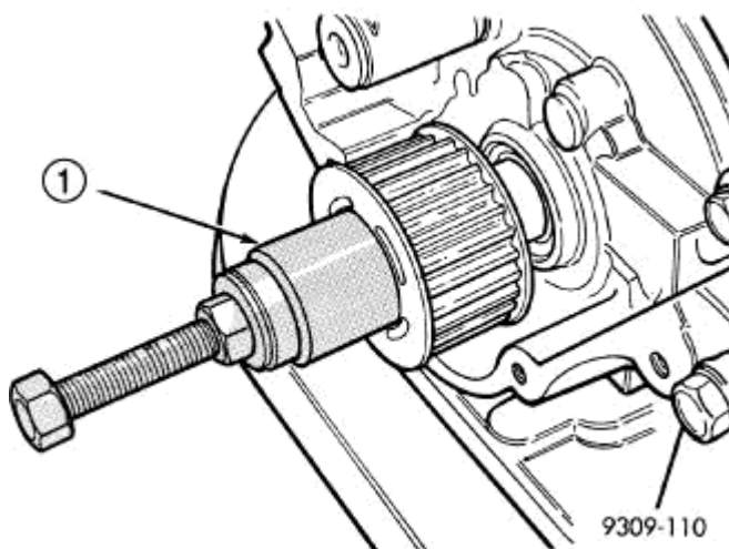
Fig. 448: Crankshaft Sprocket - Installation
