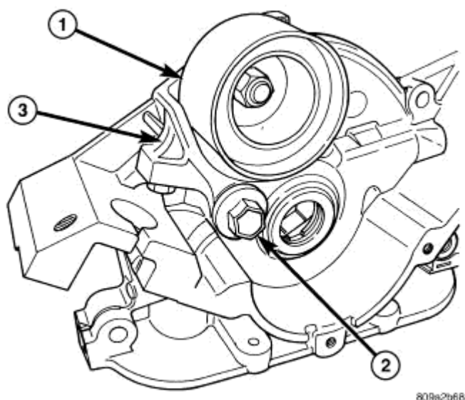
Fig. 462: TENSIONER PULLEY
