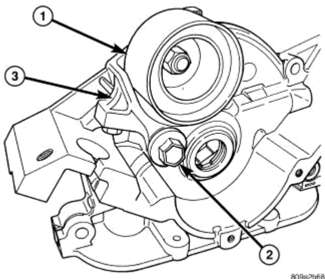
Fig. 465: TENSIONER PULLEY
