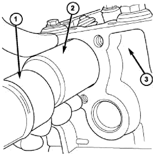
Fig. 237: CAMSHAFT SEAL
