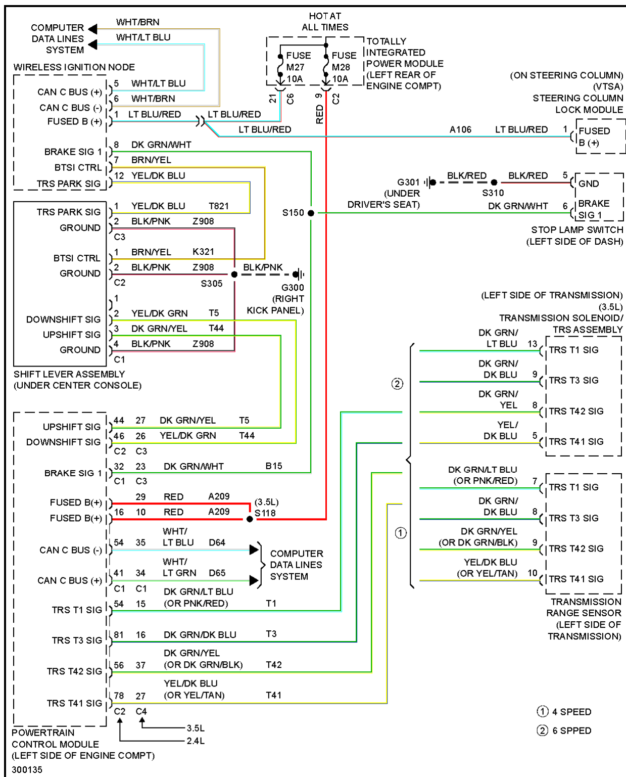
Fig. 63: Shift Interlock Circuit
