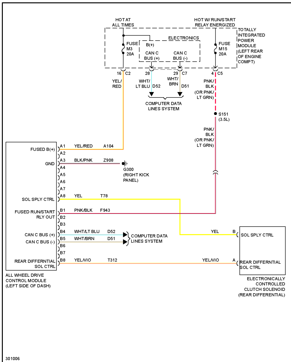
Fig. 69: AWD Circuit
